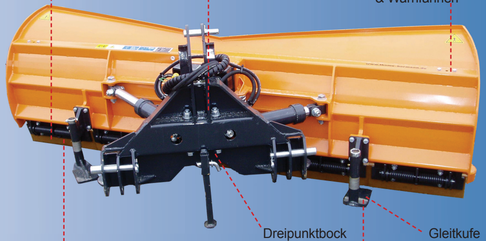
LED-Beleuchtung & Warnflaggen
