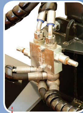
Überdruckventil
